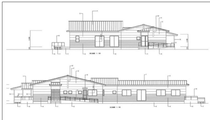
グループホームの建設予定地(アイリス北側)と 立面図。次年度4月開所予定です。
